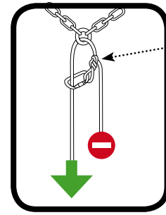
Technique de rappel sur corde à simple
